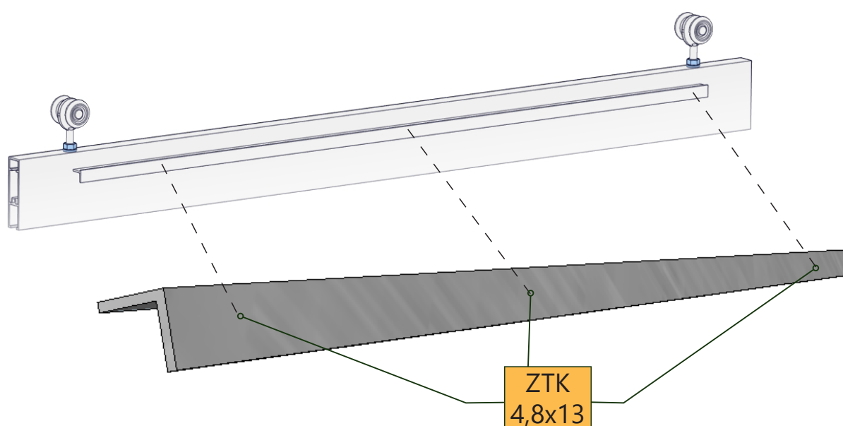
Top
